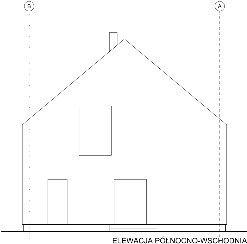
ELEWACJA PÓŁNOCNO-WSCHODNIA
