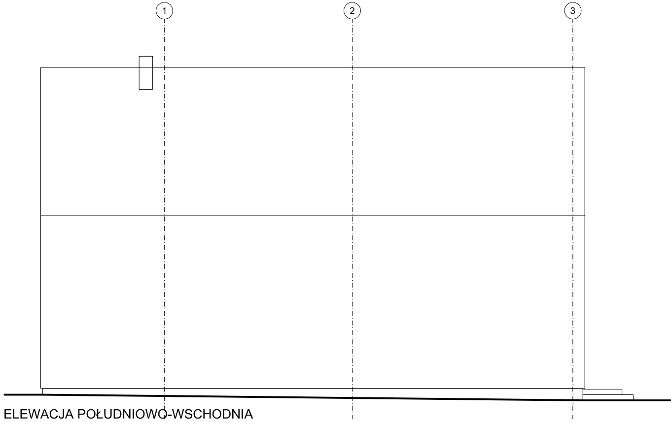
ELEWACJA POŁUDNIOWO-WSCHODNIA
