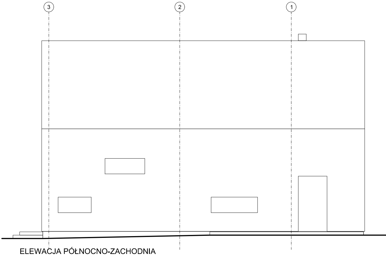
ELEWACJA PÓŁNOCNO-ZACHODNIA
